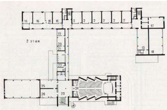
Школа № 345, 1968 г., г. Санкт-Петербург, арх. С. Евдокимов Редкая экспериментальная постройка. В школе спроектирована обсерватория, бассейн, зимний сад. У каждого класса младшей школы свой отдельный выход на улицу с собственным гардеробом
