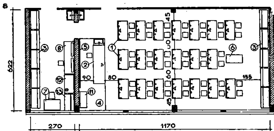
Типовая планировка старого образца для помещений лабораторий химии (А) и физики (Б). Школы и школы-интернаты. Чалдымов А.К., Степанов В.И. и др., Стройиздат, М., 1964
